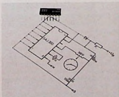
Bild 9. Integrierte Treiberschaltung SAJ 300 von ITT für quarzgesteuerte Automobiluhren
