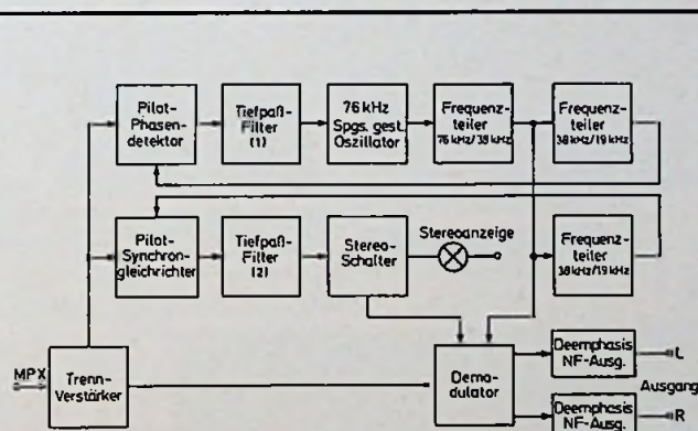
Bild 3. Blockschaltbild des Stereo-Multiplex-Dekoders \mu A 758
