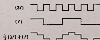
Bild 2. Verbesserte Treppenkurve
