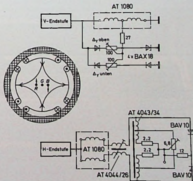
Bild 4. Schaltung zum Ausgleich von Y-Fehlern
