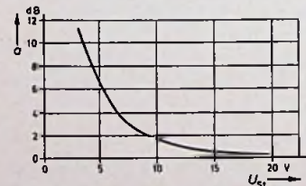
Bild 7. Abhängigkeit der Dämpfung von der Steuerungsspannung
