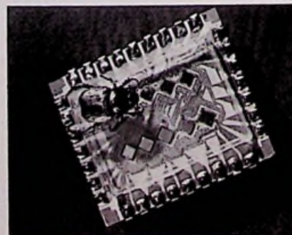
Bild 4. Durch Werkstoffwanderungen unter Streßbedingungen entstanden Aluminium-Whisker an dieser integrierten Schaltung und führten zu einem Fehler
