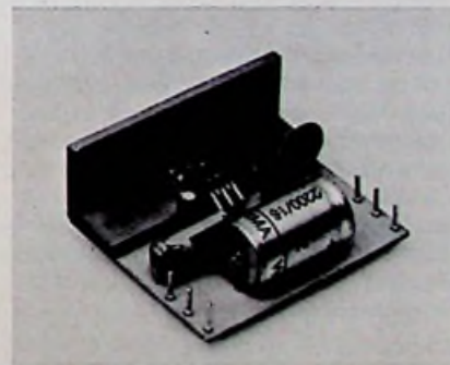
Bild 5. Der 7-W-Verstärker mit der L 140 von SGS-Ates kommt mit sehr wenigen zusätzlichen Bauelementen aus
