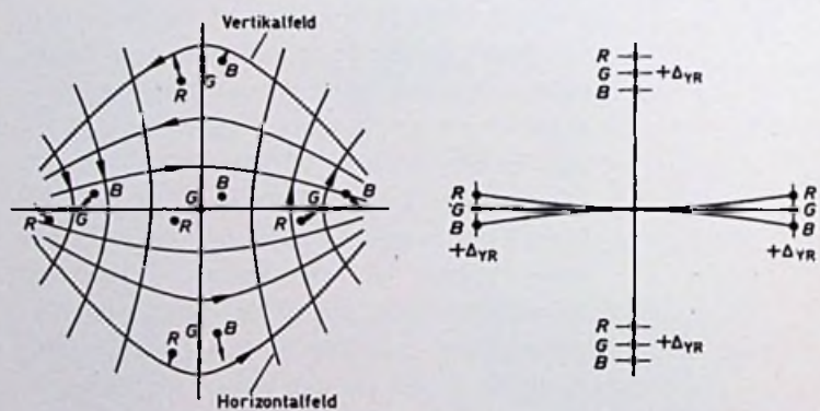
Bild 1. Fehler bei Verdrrehung der Strahlerzeugungssysteme
