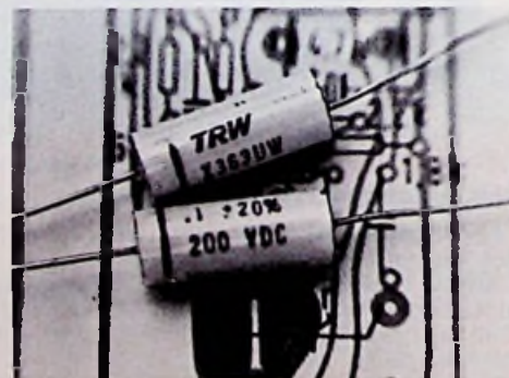
Kondensatoren aus metallisiertem Polypropylen (Foto: TRW)
