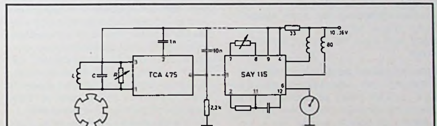
Bild 11. Die Tachometerschaltung SAY 115 von Sescosem kann über Frequenzteiler den Schrittmotor eines Tages-Kilometerzählers steuern
