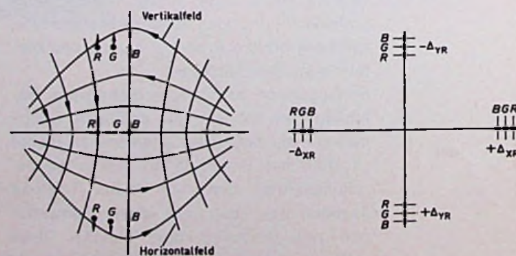
Bild 2. Fehler bei seitlichem Versatz der Strahlensysteme
