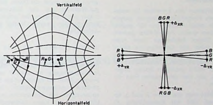
Bild 3. Fehler bei vertikalem Versatz der Strahlerzeugungssysteme
