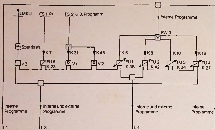
Bild 2. Kopfstation für Schultonrundfunk-Programme, 3 externe und 4 schulinterne Fernseh-Programme zu einem Zweifelhernetz (Bild: Hirschmann)
