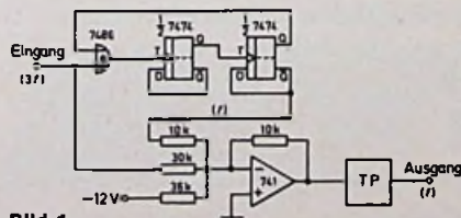
Bild 1. Schaltung eines digitalen Frequenzteilers
