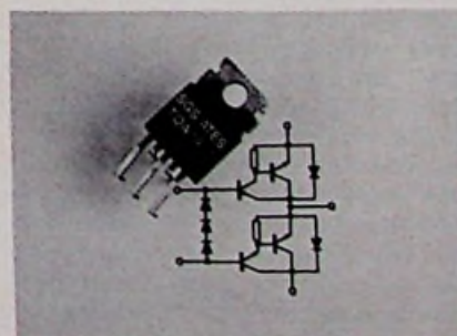
Bild 6. Dieser quasicomplementäre Endverstärker von SGS-Ates ist für Nennspannungen von 36 V und 46 V erhältlich
